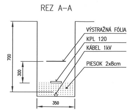
DETAIL ULOŽENIA KÁBLOV
