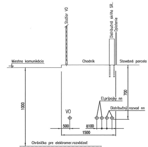
DETAIL ULOŽENIA KÁBLOV
