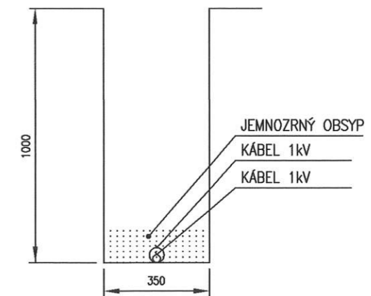
REZ A-A
